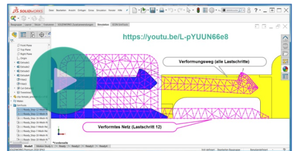
Abbildung 2: Verformungswege exportieren
